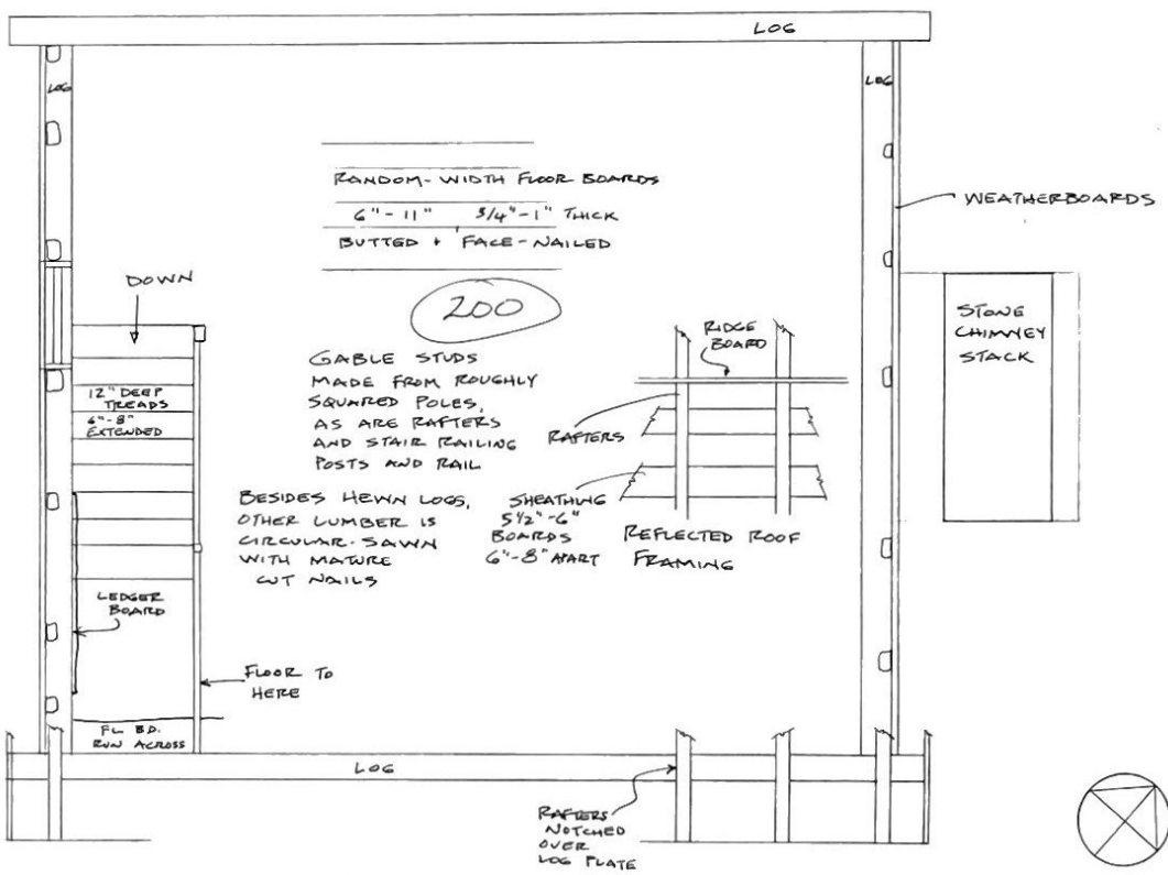
LOFT PLAN
