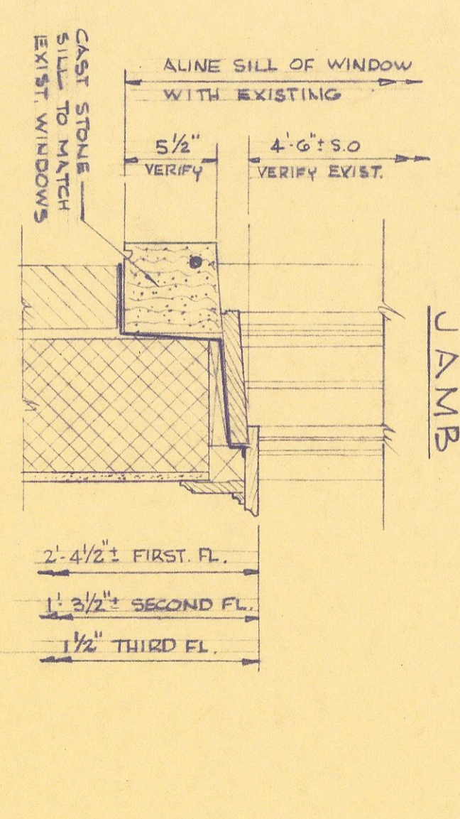
JAMB
